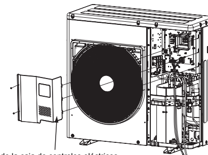
Tapa de la caja de controles eléctricos
