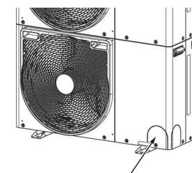
Prepunzonado para los cables de comunicación y los tubos de refrigerante
