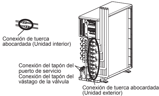
* Ejemplo de punto de comprobación (RAS-5M34G3AVG-E)
