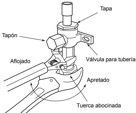
Válvula del lateral del gas
