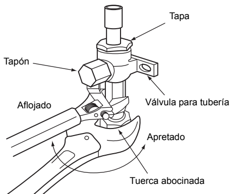
Válvula del lateral del gas
