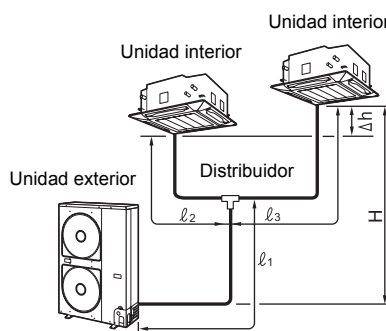
Ejemplo de sistema simultáneo gemelo
