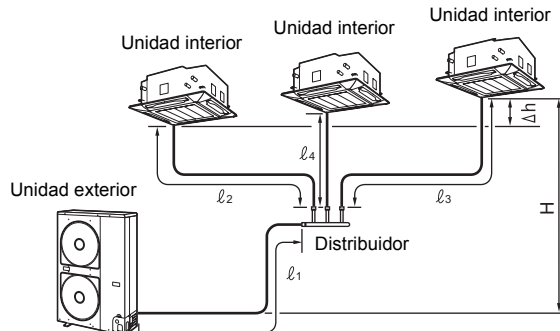
Ejemplo de sistema simultáneo triple
