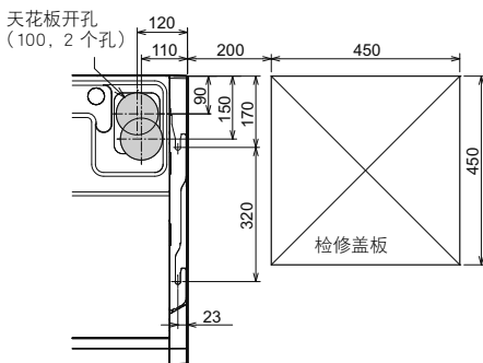
天花板开孔的位置
