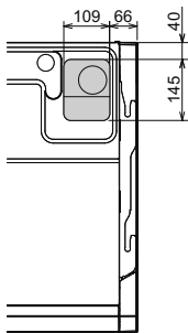
Θέση της σπής απόσπασης στο άνω μέρος της εσωτερικής μονάδας
