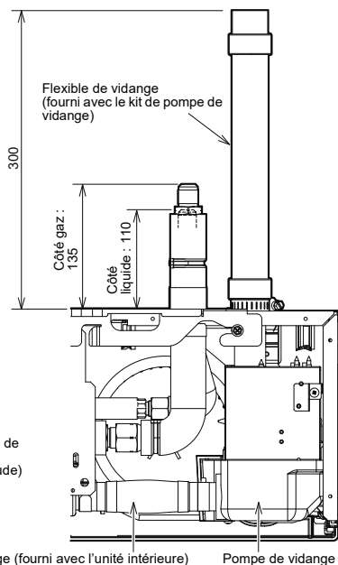
Position des conduites de réfrigérant et de la conduite de vidange
