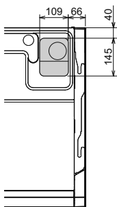
Posição pre-cortada no topo da unidade interior
