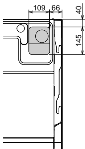
室内机顶部顶出孔板的位置
