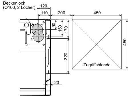
Position des Deckenlochs
