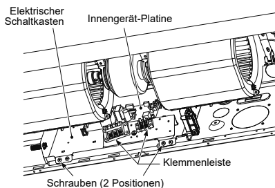
Position der Anschlüsse auf der Innengerät-Platine
