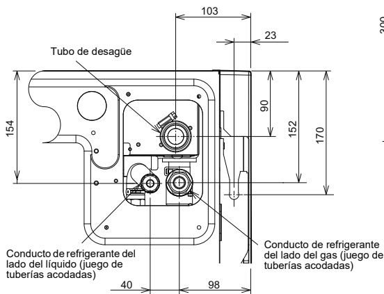
Posición de los conductos de refrigerante y tubo de desagüe
