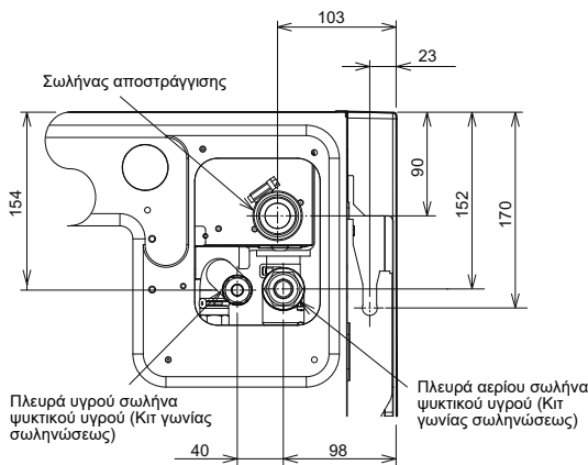
Θέση των σωλήνων ψυκτικού υγρού και του σωλήνα αποστράγγισης
