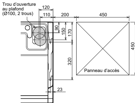
Position du trou d'ouverture au plafond
