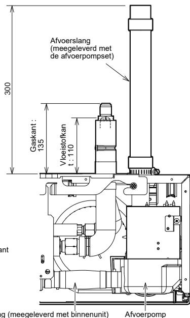
Positie van koelmiddelleidingen en afvoerleiding
