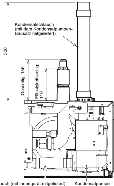
Position der Kühlmittelleitungen und des Ablaufrohrs
