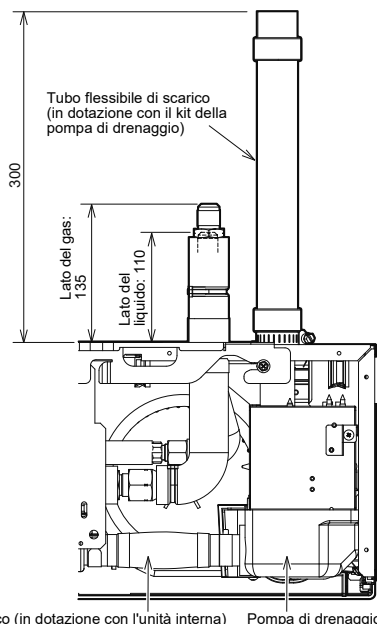
Posizione dei tubi del refrigerante e del tubo di scarico
