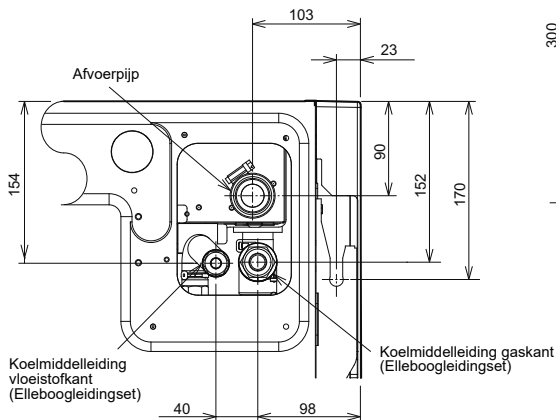
Positie van koelmiddelleidingen en afvoerleiding
