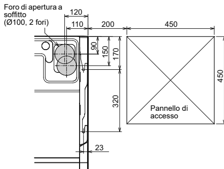
Posizione del foro di apertura a soffitto
