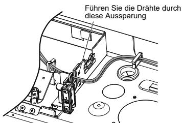
Position der Anschlüsse auf der Innengerät-Platine
