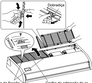
Botão de fixação da grelha de admissão de ar Grelha de admissão de ar
