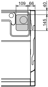
Position der vorgeprägten Öffnung an der Oberseite des Innengeräts
