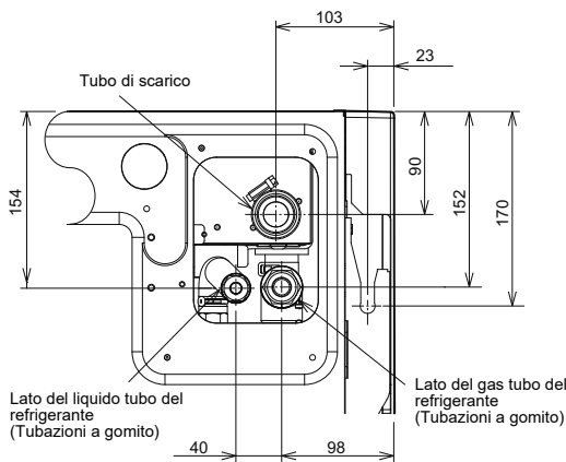
Posizione dei tubi del refrigerante e del tubo di scarico
