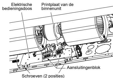
Positie van aansluitingen op printplaat binnenunit
