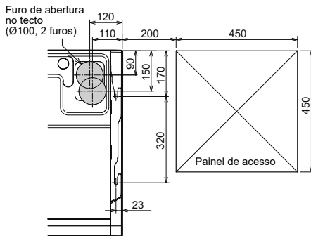
Posição do orifício de abertura no tecto
