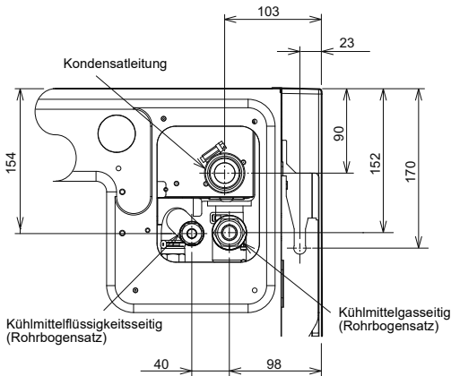
Position der Kühlmittelleitungen und des Ablaufrohrs
