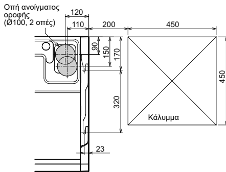
Θέση της σπής ανοίγματος οροφής
