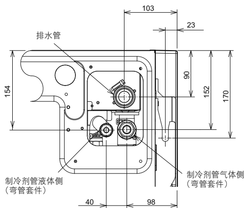
制冷剂管和排水管的位置
