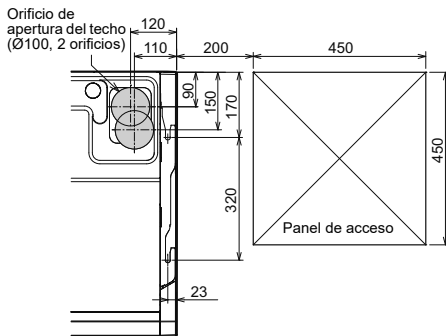
Posición del orificio de apertura del techo
