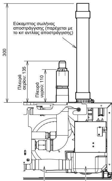
Θέση των σωλήνων ψυκτικού υγρού και του σωλήνα αποστράγγισης
