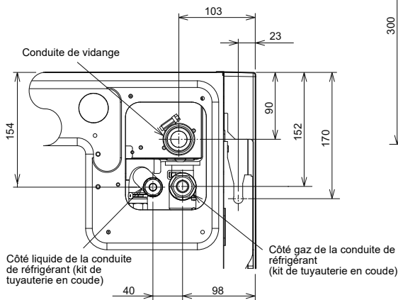
Position des conduites de réfrigérant et de la conduite de vidange
