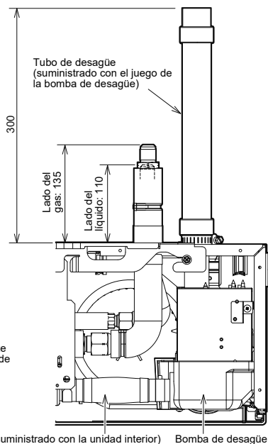
Posición de los conductos de refrigerante y tubo de desagüe
