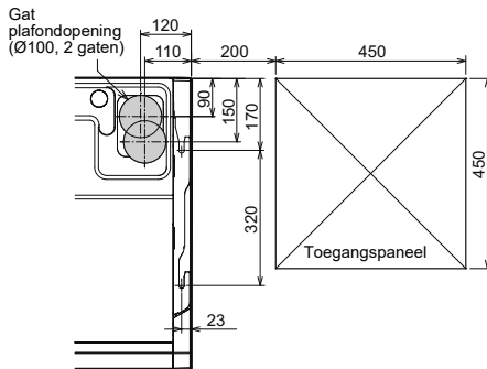
Positie van gat plafondopening
